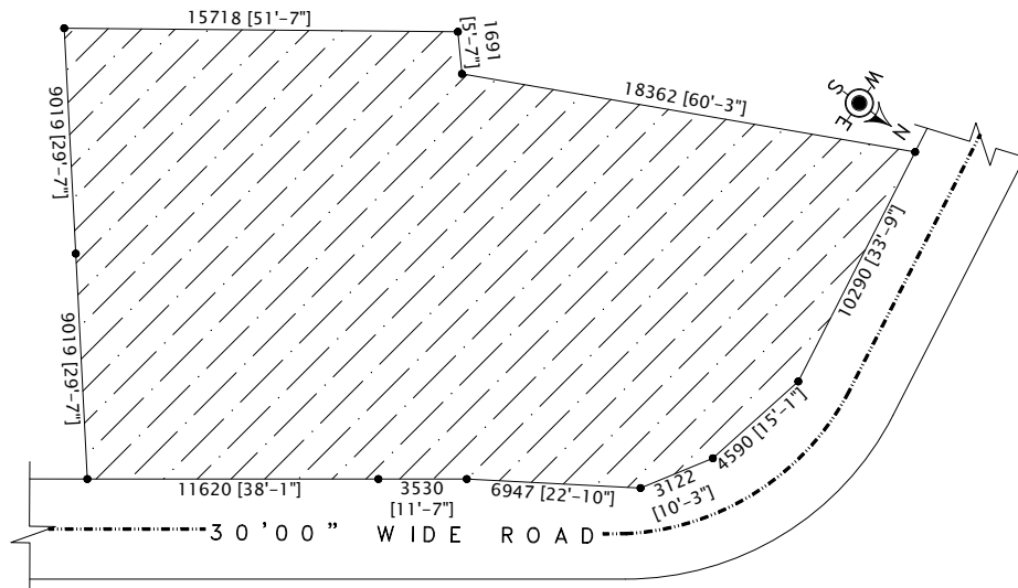
(J) LAYOUT MAP SCALE: 1:200
